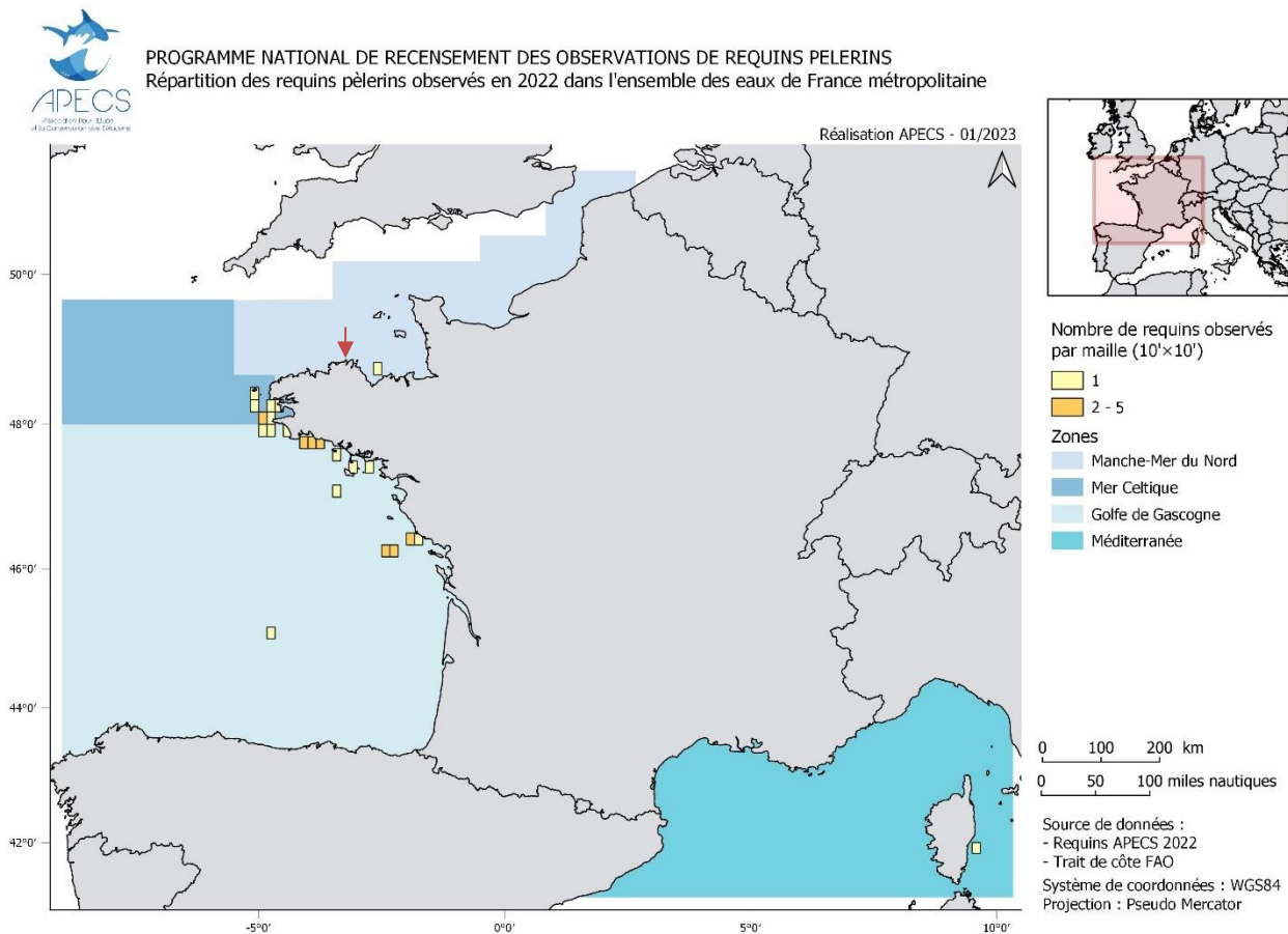
Figure 5 : Répartition spatiale des requins pélerins observés en France métropolitaine en 2022
