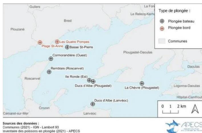
Carte des sites de plongée inventoriés sur une journée. I APECS
